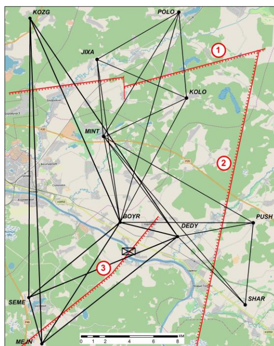
Рисунок 2. Схема геодезической сети ГДП «Полоцкая ГЭС» и тектонические разломы ☒ - Полоцкая ГЭС; ———— - тектонические разломы: ① - Полоцкий; ② - Чашникский; ③ - Туровлянский
