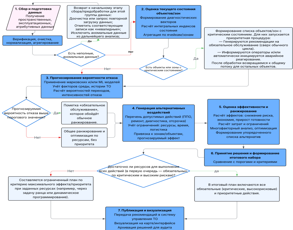
Рисунок 4.4 – Блок-схема алгоритма адаптивного управления техническим обслуживанием COMM и ИТСО
