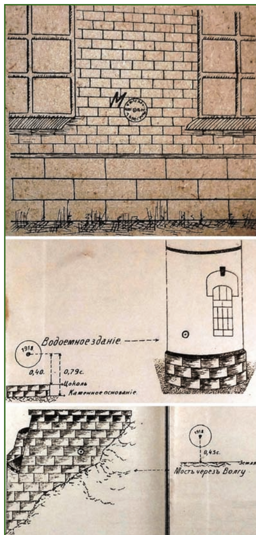
Рис. 3 Размещение нивелирных марок в зданиях и сооружениях [6]
